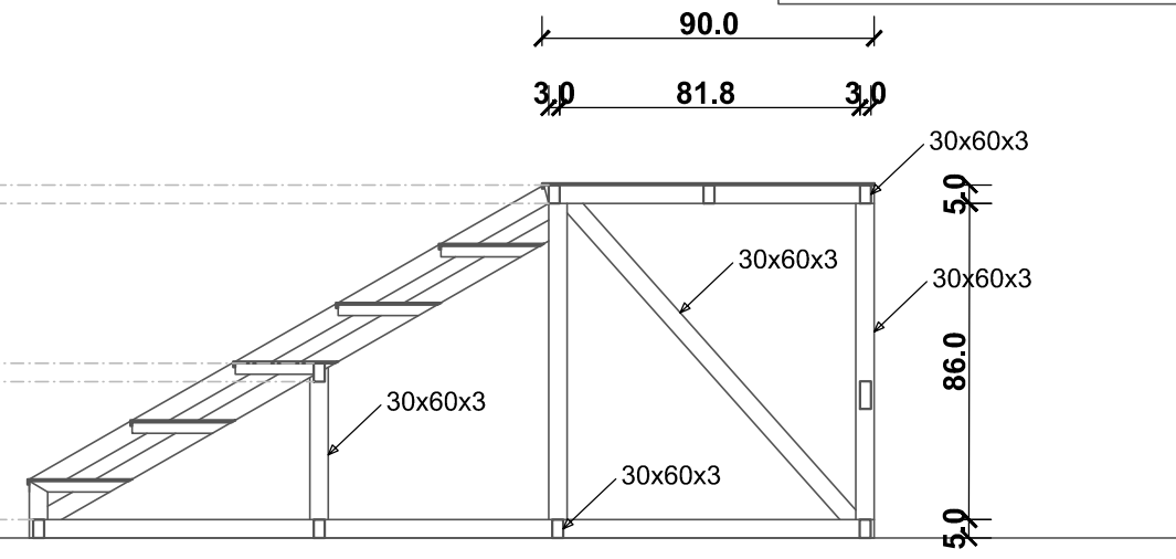
ПРЕСЕК А-А СТЕПЕНИШТА 4
